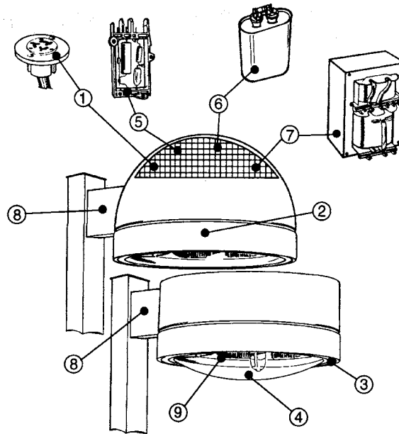
DECASPHERE™ LUMINAIRE
